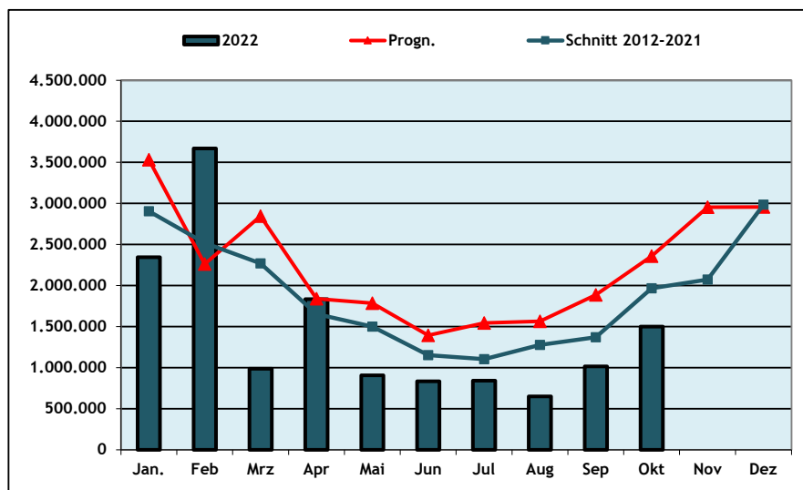
Übersicht der monatlichen Brutto-Erträge in kWh
