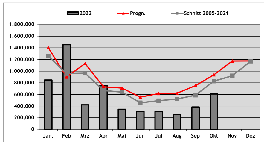
Übersicht der monatlichen Brutto-Erträge in kWh
