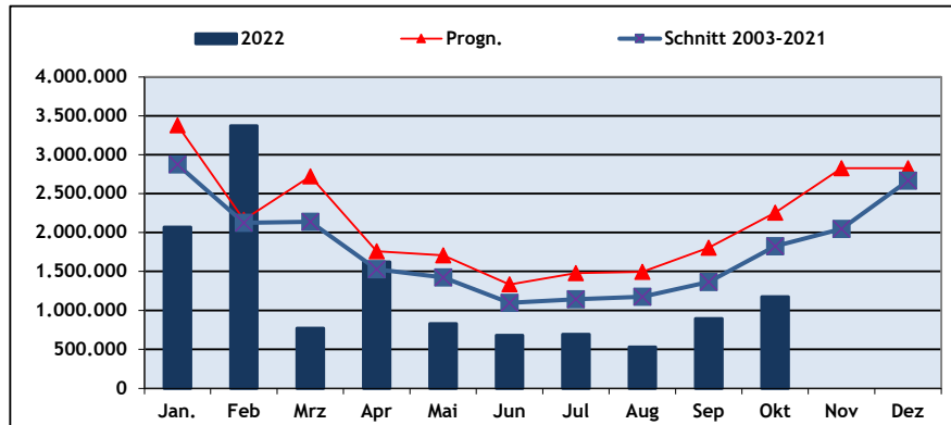
Übersicht der monatlichen Brutto-Erträge in kWh
